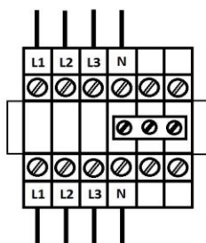
Рис.5 Подключение электрического котла к трехфазной сети
