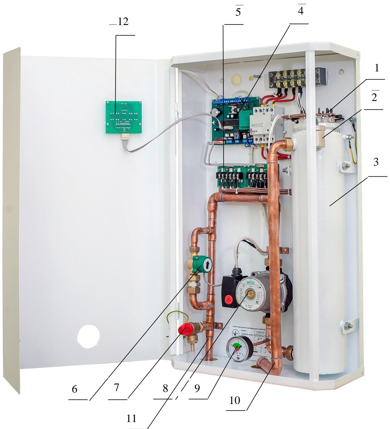
Рис.1 Конструкция трехфазного котла серии «Comfort -24,0»
